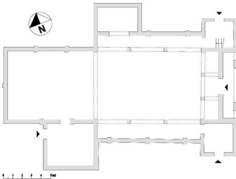
Ryc. 9. Mochowo, kościół pw. św. Marcina, rzut przyziemia
