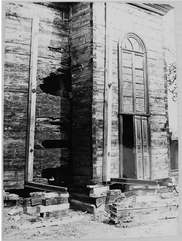
Ryc. 13. Mochowo, kościół pw. św. Marcina, widok od południa – zniszczenia belek ścian korpusu nawowego przy styku z wieżą, po zdjęciu zewnętrznego szalunku
